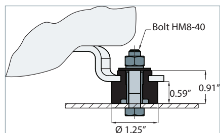
Silent bloc
