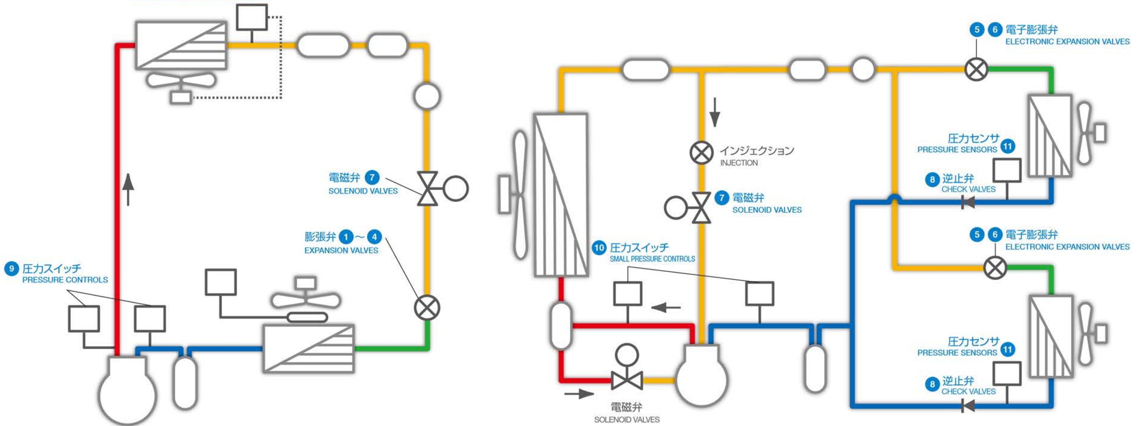
12 ファンスピードコントローラ CONDENSER FAN SPEED CONTROLS
