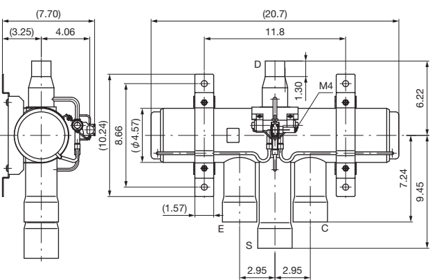
Type STF-60U9G
