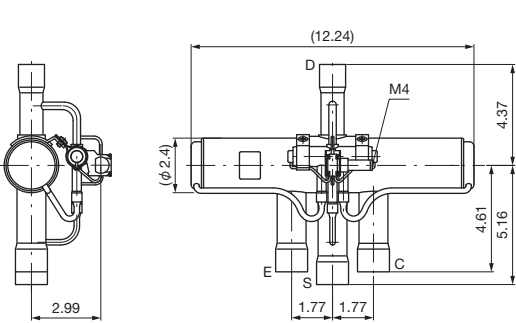
Type STF-25U22G
