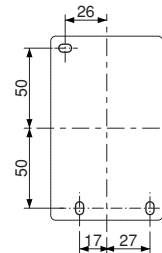
壁取付寸法
