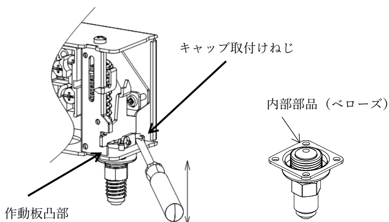
圧力スイッチ高圧側
