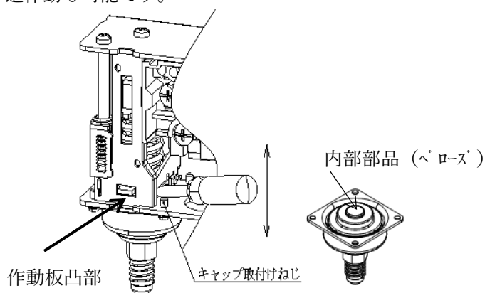
圧力スイッチ低圧側
