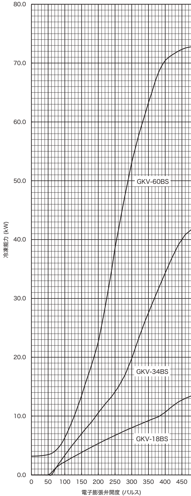
R410A 能力表
