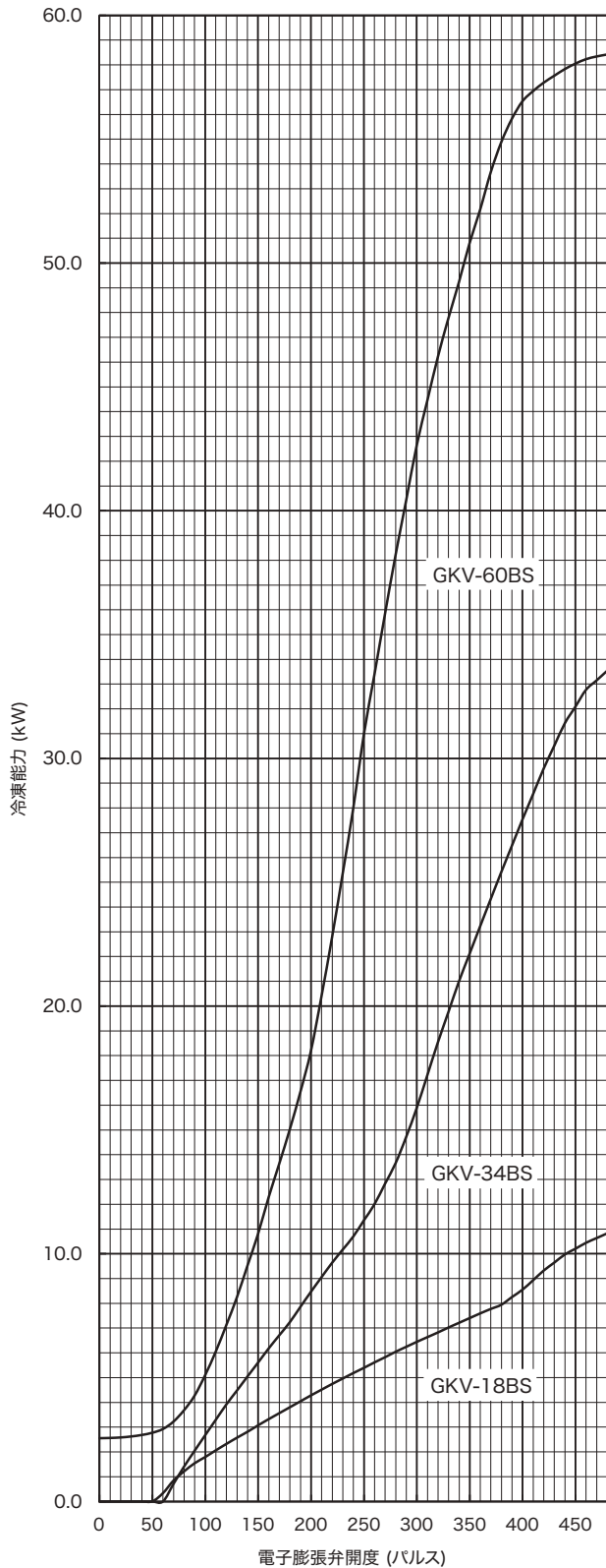
R449A 能力表
