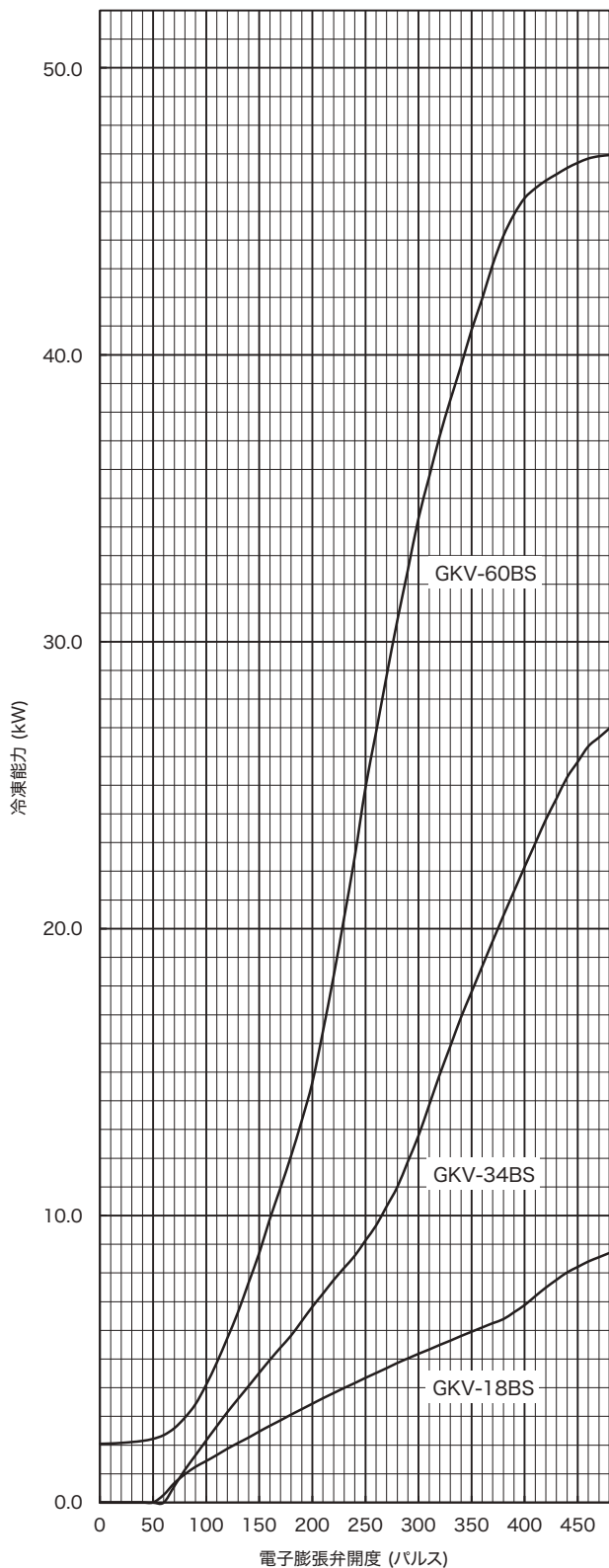
R134a 能力表
